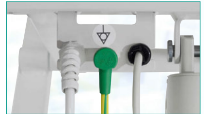
Potenzialausgleichkabel (zwingend erforderlich bei Anwendung „interkardiales Verfahren“)
